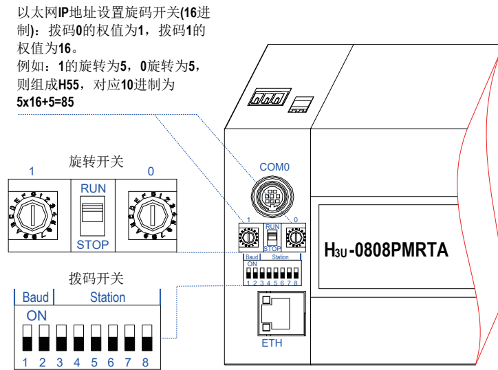
H 3U -3624MT/R、H 3U -3232MT/R、H 3U -0808PMRТА 的以太网通信接口示意图
