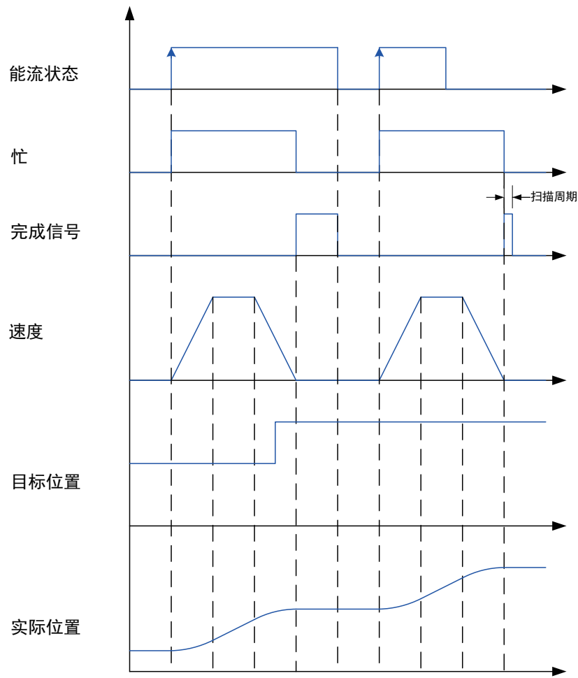
MCMOVABS 时序图
